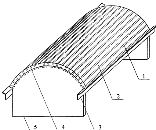
1 – шпильцы (заполнить шпаклевочной смесью); 2 – ГКЛ с параллельными пазами; 3 – опора для ГКЛ (уголок); 4 – лицевая сторона; 5 – шаблон
