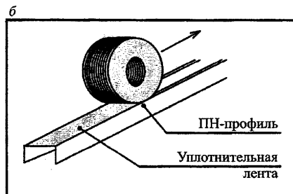
а – разметка положения перегородки на полу; б – наклеивка уплотнительной ленты на профиль каркаса
