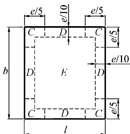
ПЛАН КРОВЛИ
