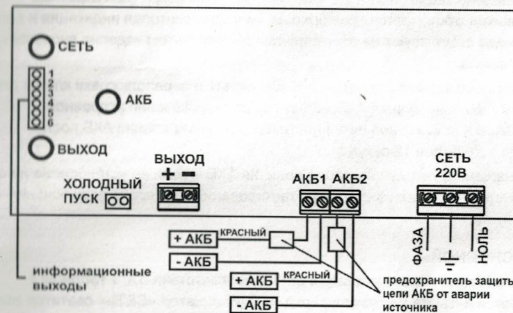
Рисунок 1 - вид изделия с открытой крышкой
